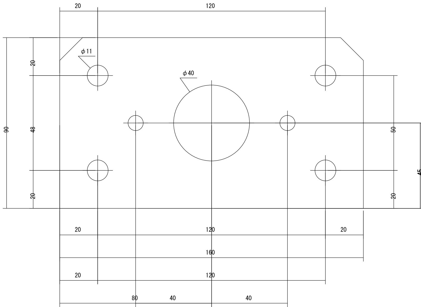
正面図
